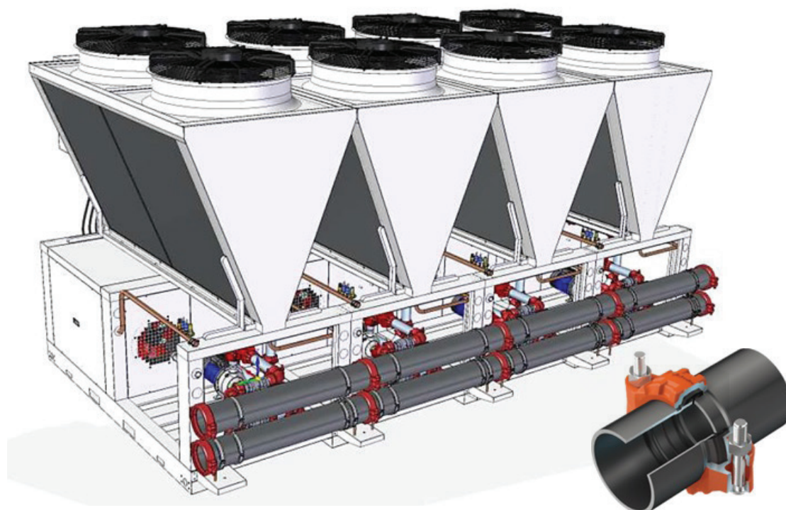
Dessin 10 : Collecteur hydraulique à l'arrière des appareils en cascade
