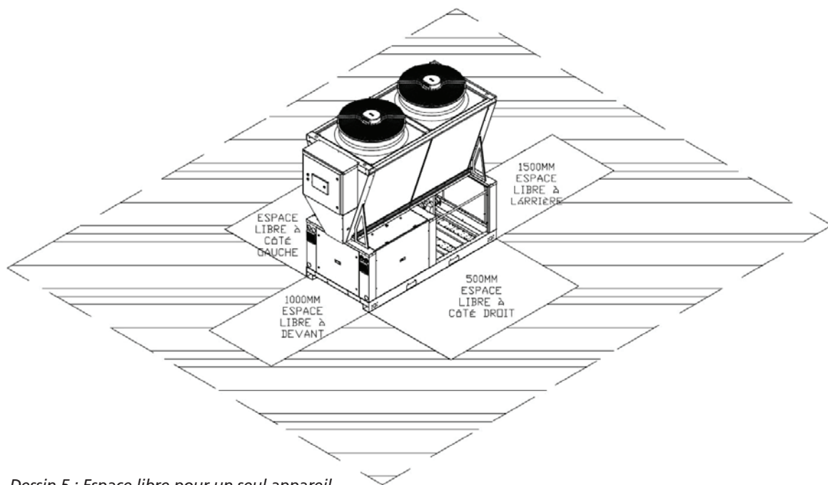
Dessin 5 : Espace libre pour un seul appareil
