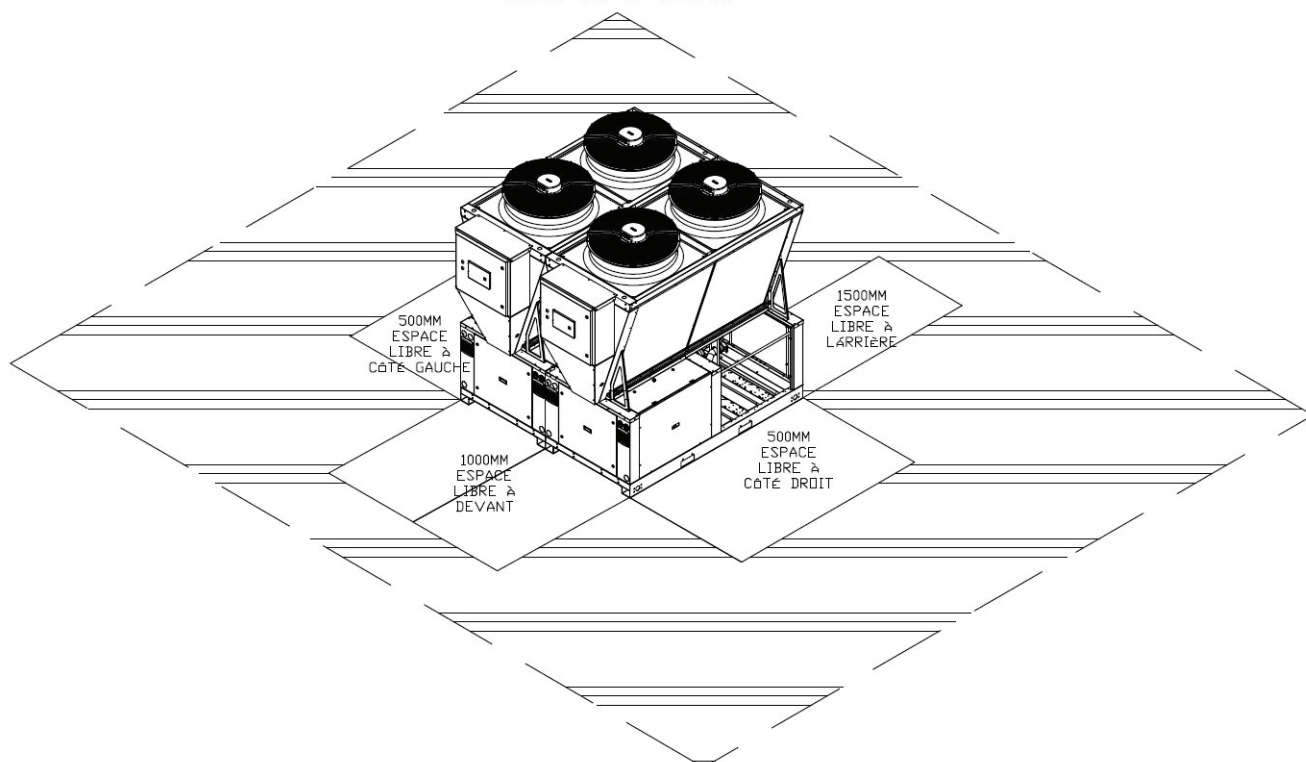
Dessin 6 : Espace libre pour plusieurs appareils
