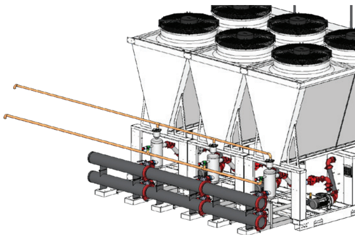
Dessin 7 : Dégazeurs installés entre les appareils et les tuyaux de raccordement
