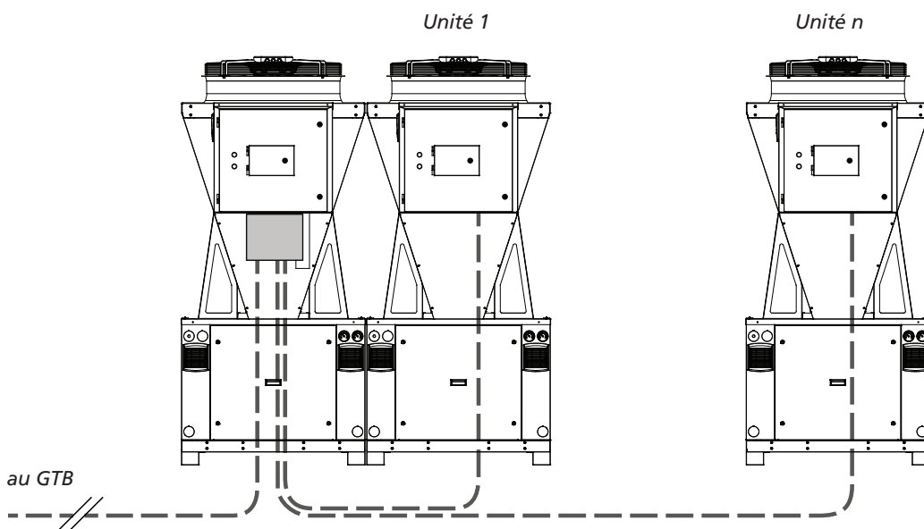
Dessin 15 : Câblage en cascade
