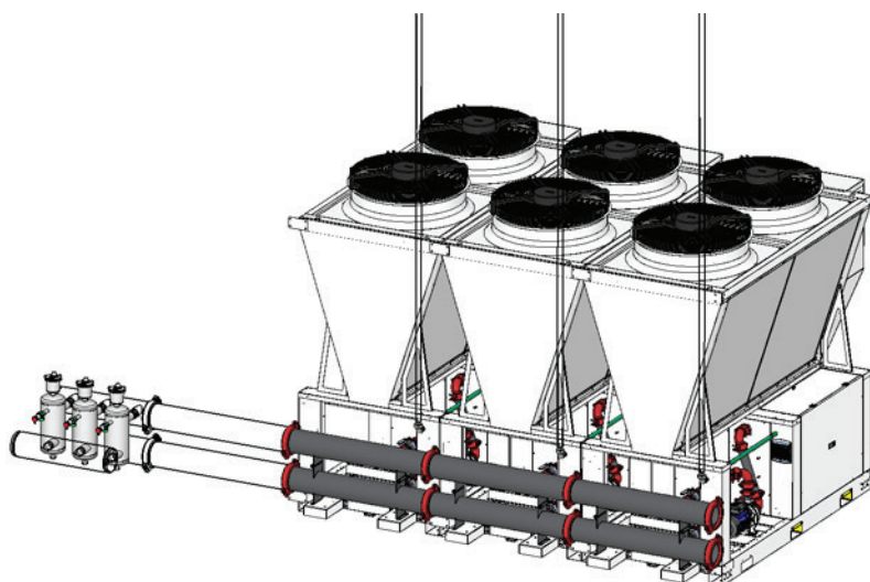
Dessin 8 : Dégazeurs montés à distance de l'équipement
