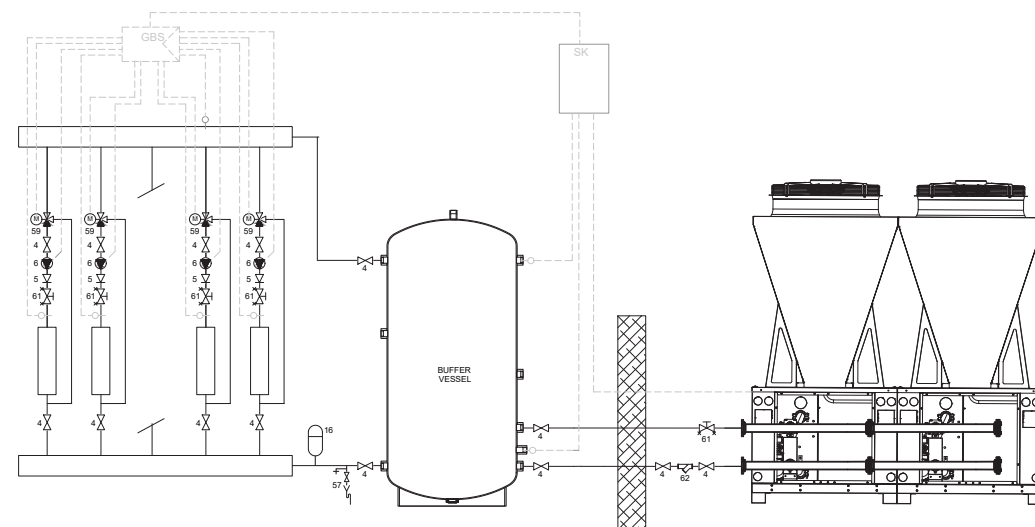
Dessin 11 : Enevator Altus pour le chauffage des locaux
