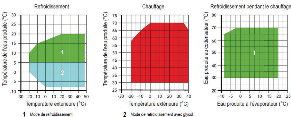
Dessin 17 : Limites de fonctionnement Appareil 4 tubes
