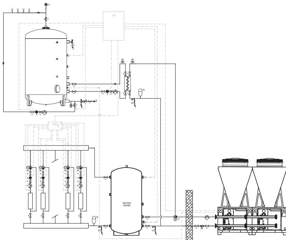
Dessin 13a : Enevator Altus pour le chauffage des locaux et la préparation de l'eau chaude sanitaire*
