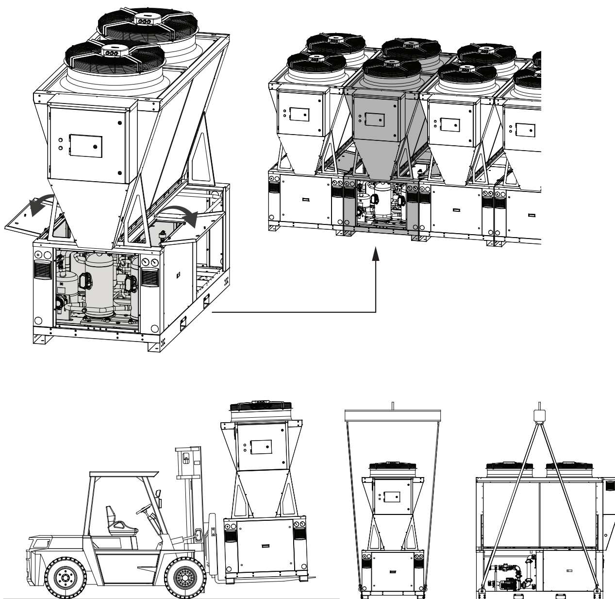
Dessin 3 : Points de levage
