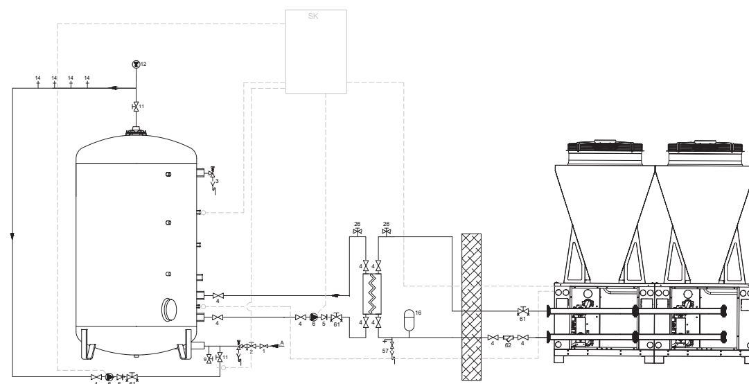
Dessin 12 : Enevator Altus pour la préparation d'eau chaude sanitaire
